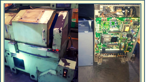
ติดตั้ง Inverter CNC นานู โนเดอเก่า
