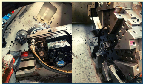
Overhaul Turret CNC SYD PL15
